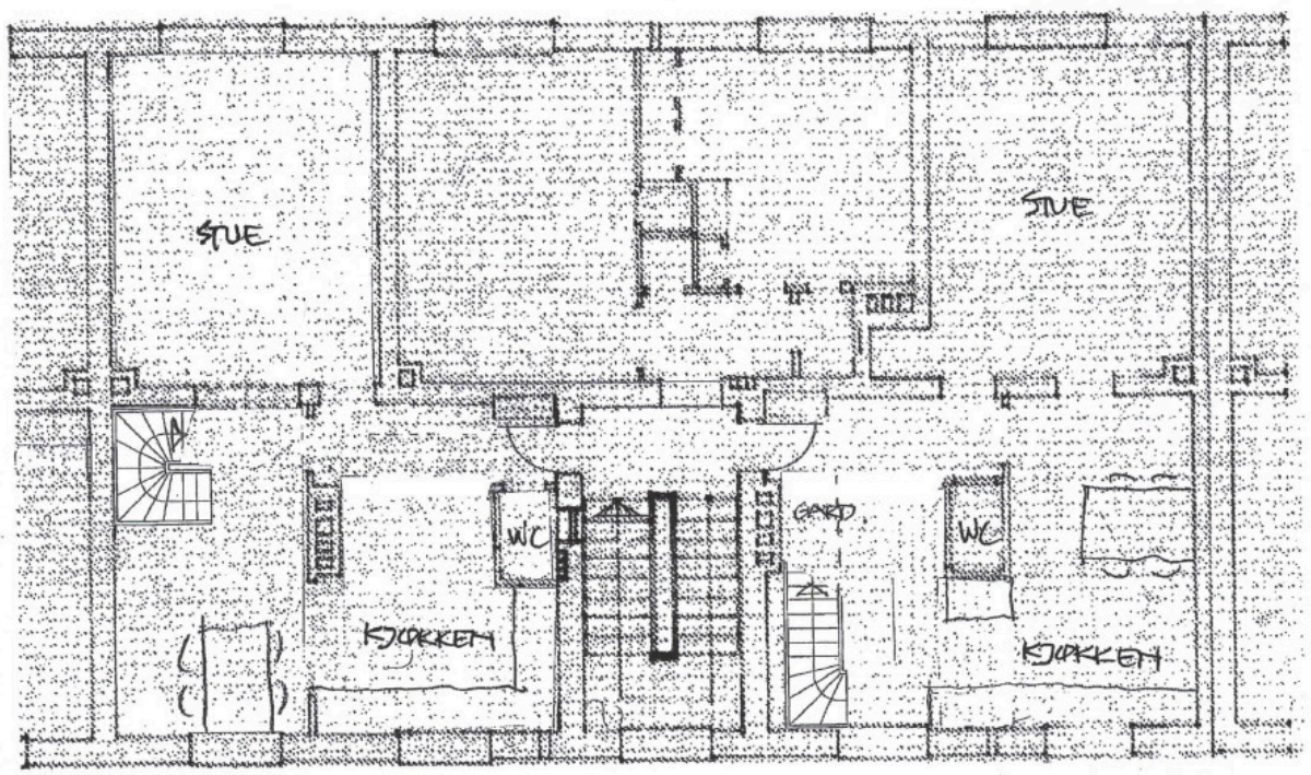
3. etasje
